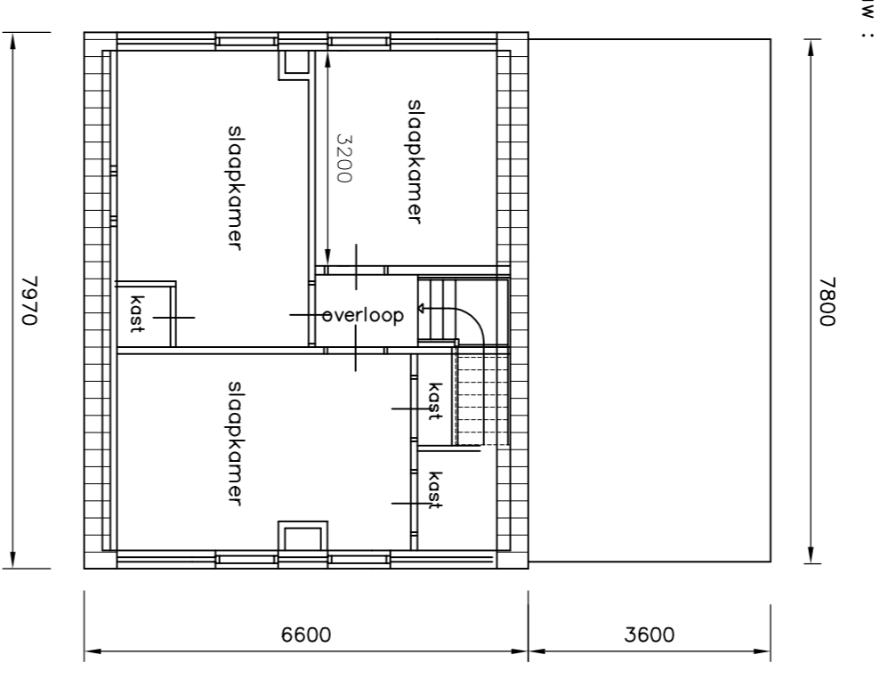
VERDIEPING BESTAAND
