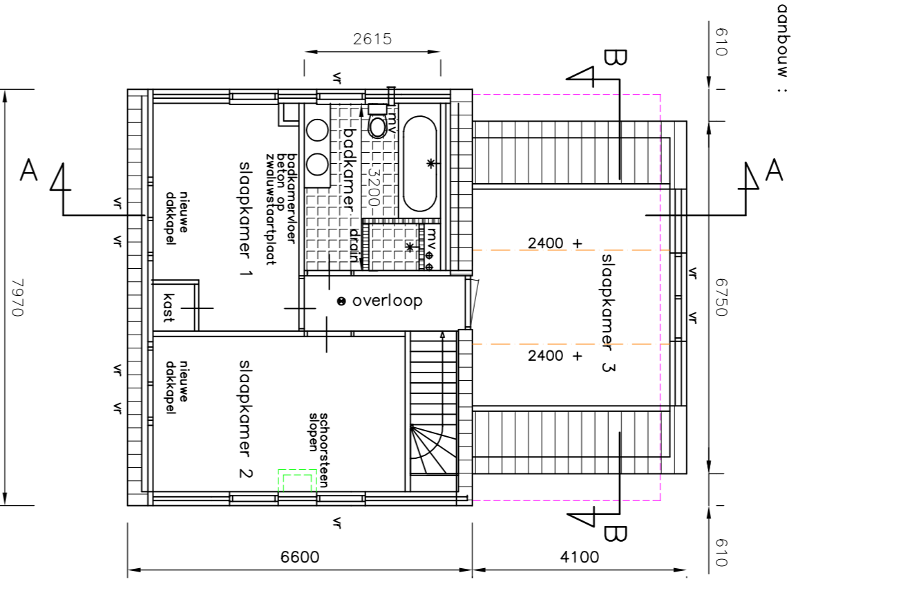
VERDIEPING GEWUJZIGD
