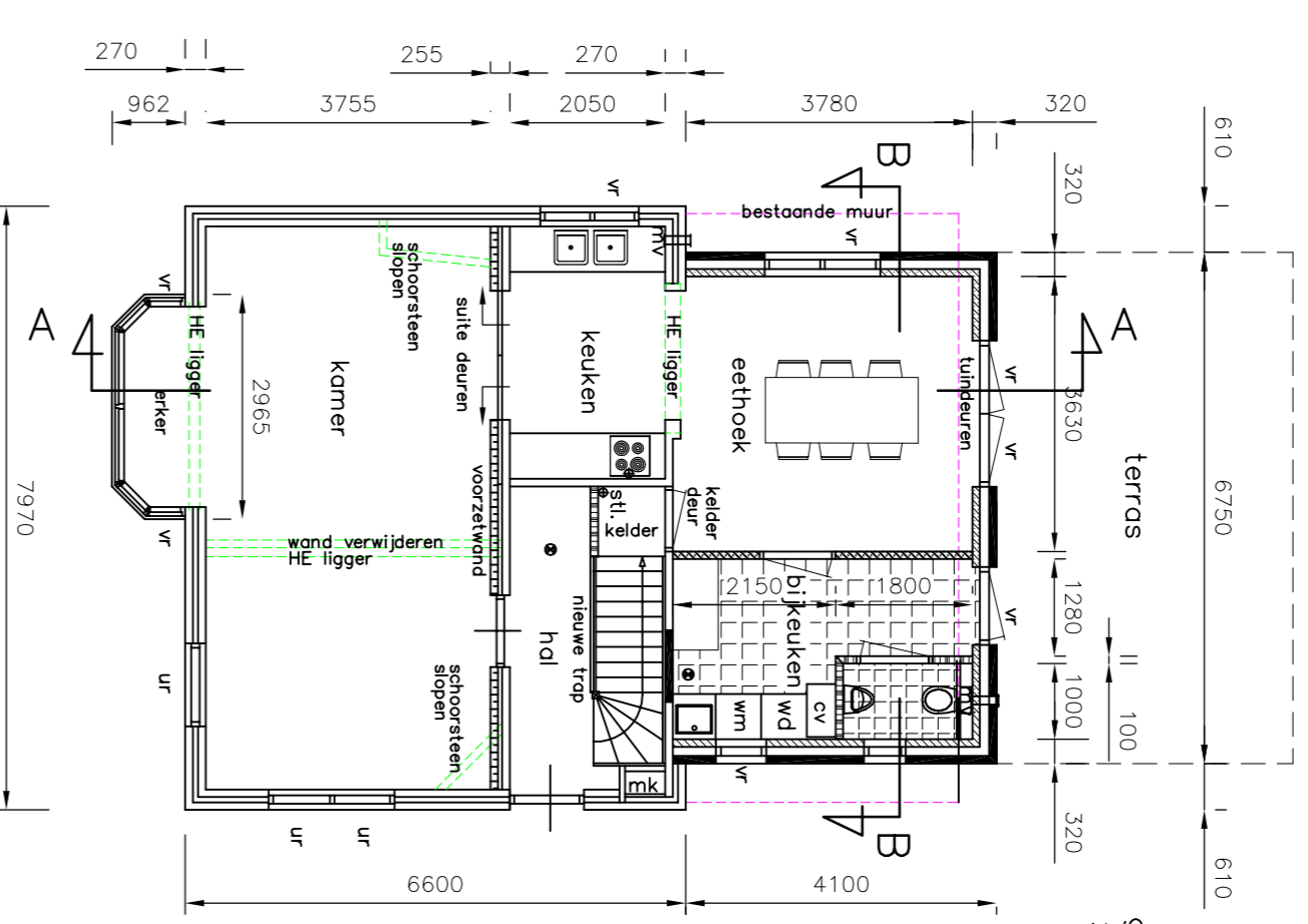
BEGANE GROND GEWUJZIGD
